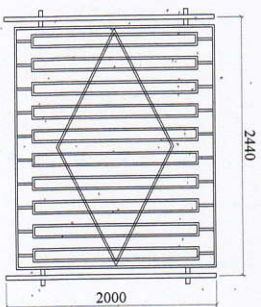
Эскиз проектируемой секции ограждения
